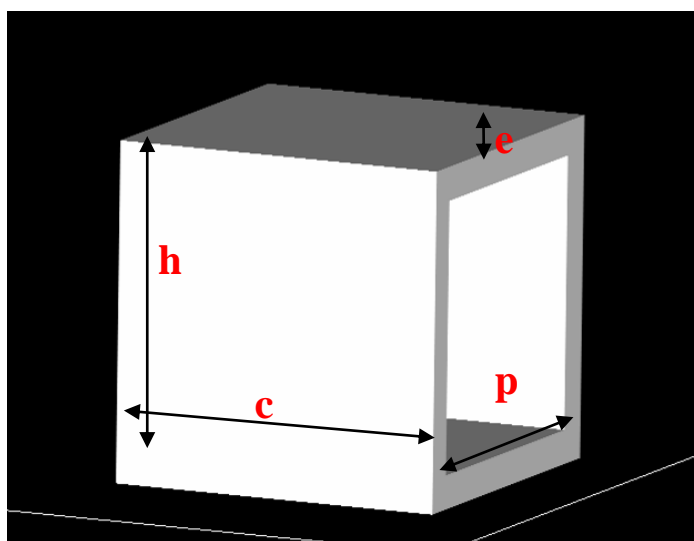
Figura 8. Croqui esquemático das dimensões dos blocos estudados
